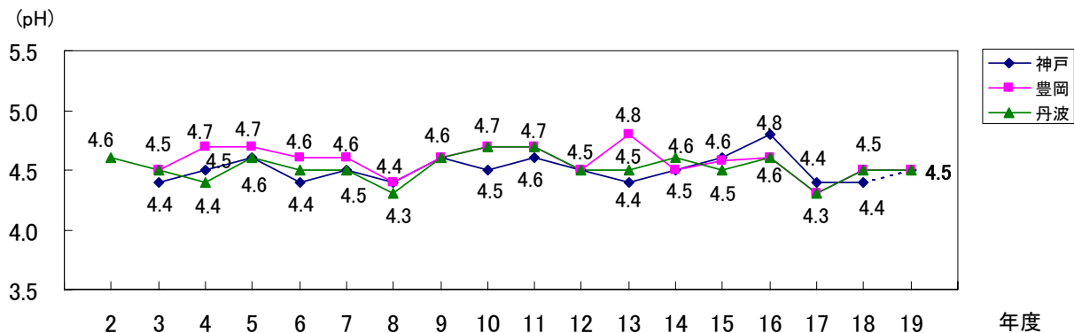
図4 酸性雨自動測定機によるpH監視測定結果
