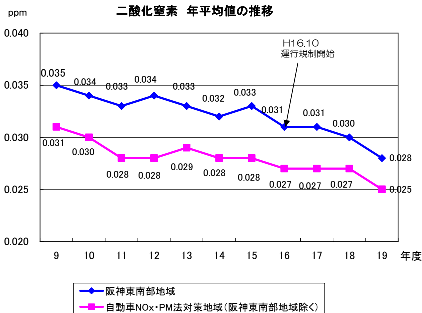
図7 自動車NOx・PM法対策地域の環境濃度の推移
