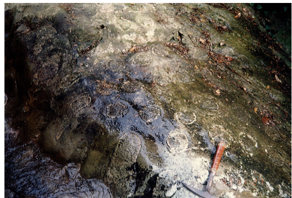
溶結凝灰岩中の2次噴気孔
