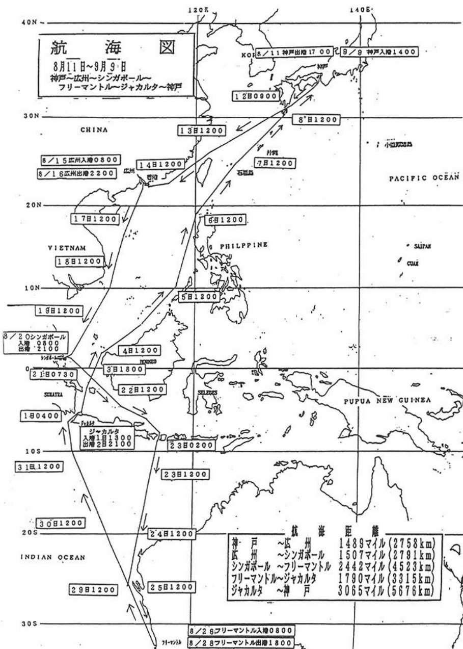
第2-5-16図 航海図
