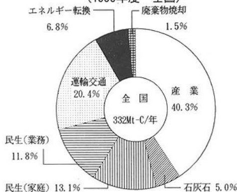
第2-5-8図 二酸化炭素排出量
