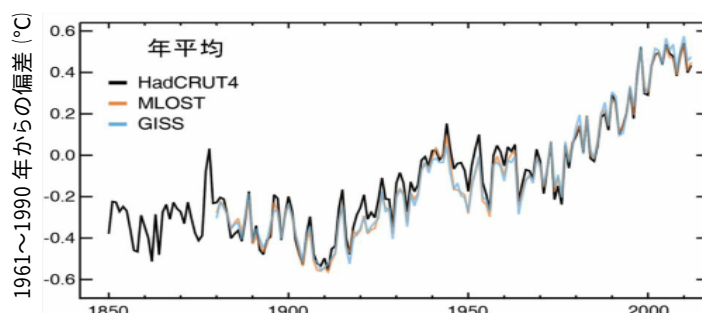
世界の地上気温の経年変化
