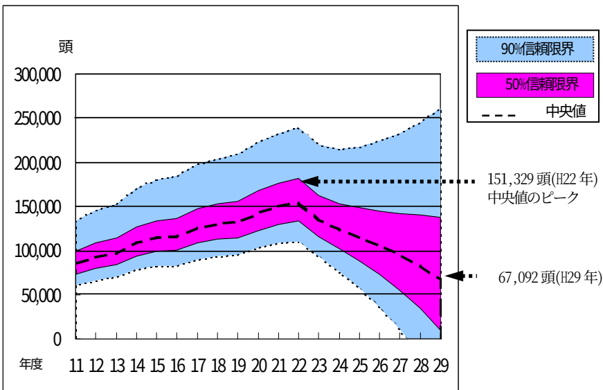
第3-2-4図 シカ推定生息数の推移(全県)
