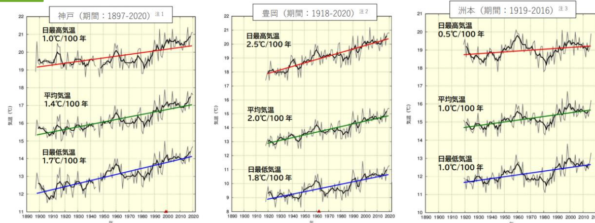
県内の気温の推移
