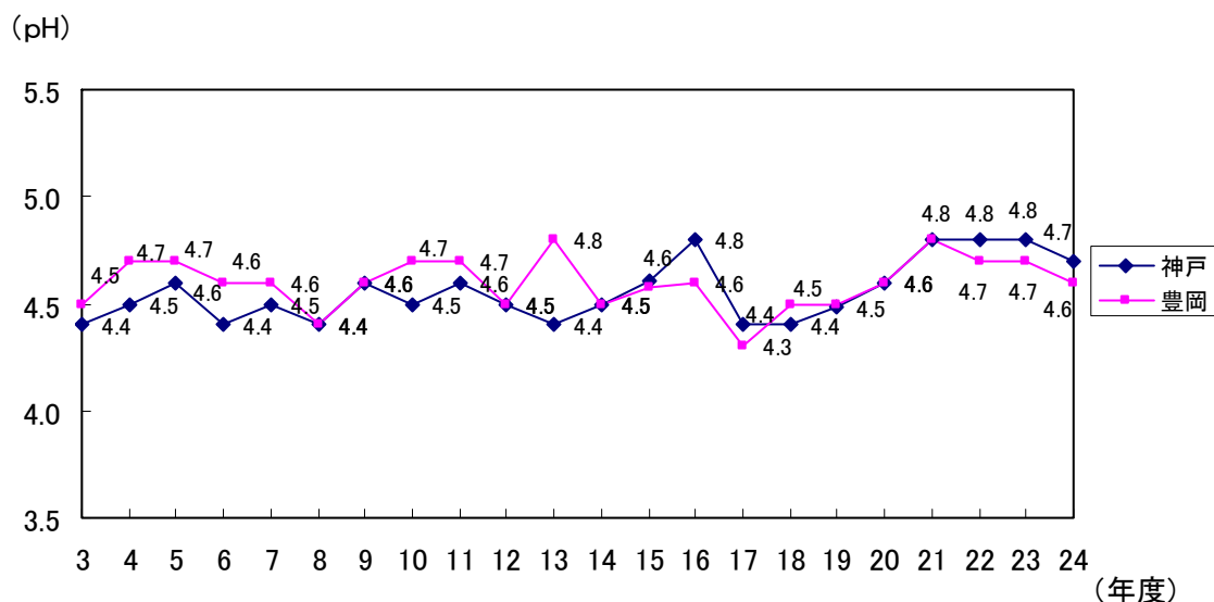
図6 雨水のpHの推移
