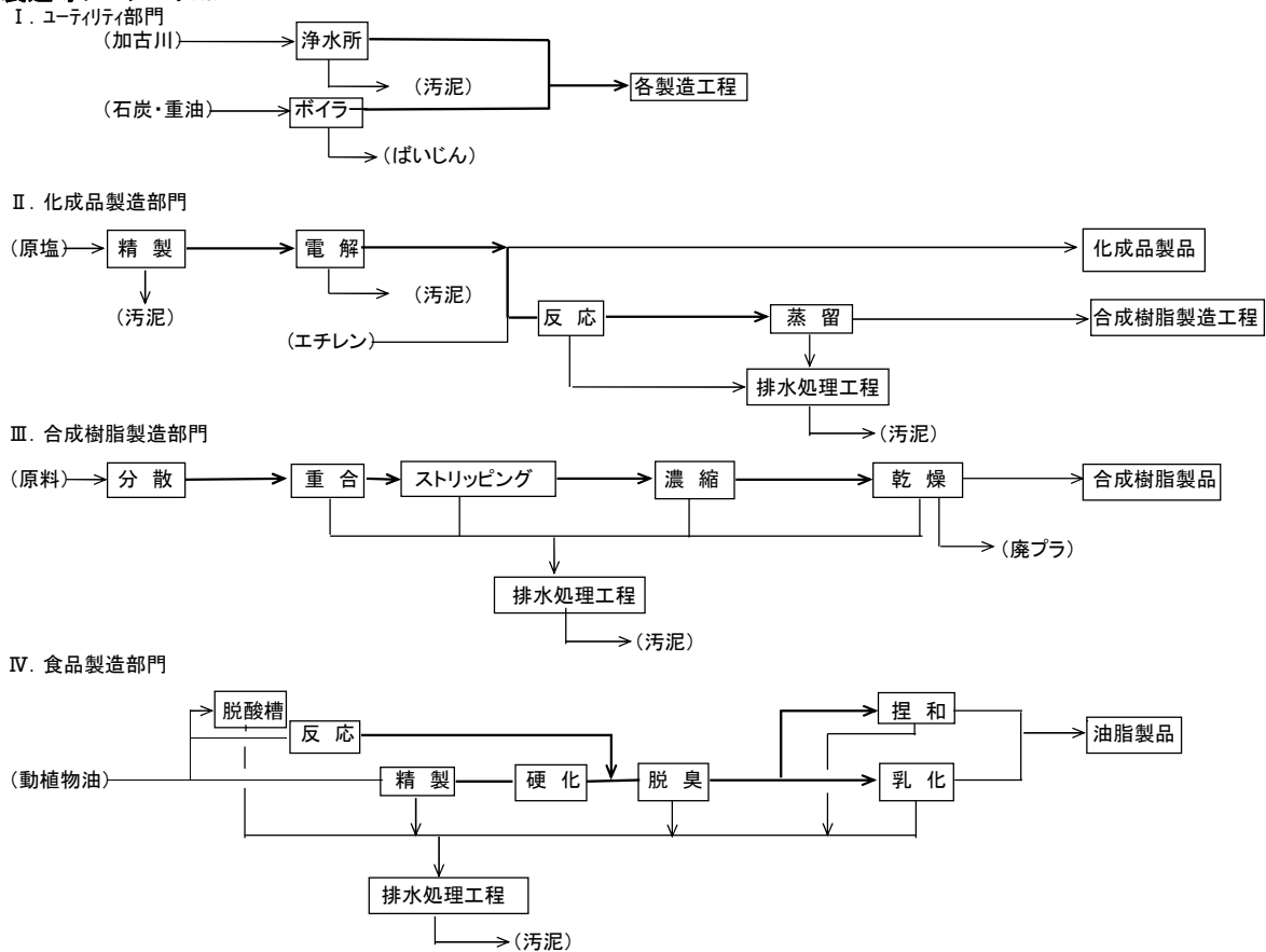
図-1: 製造等フロシートNo.1
