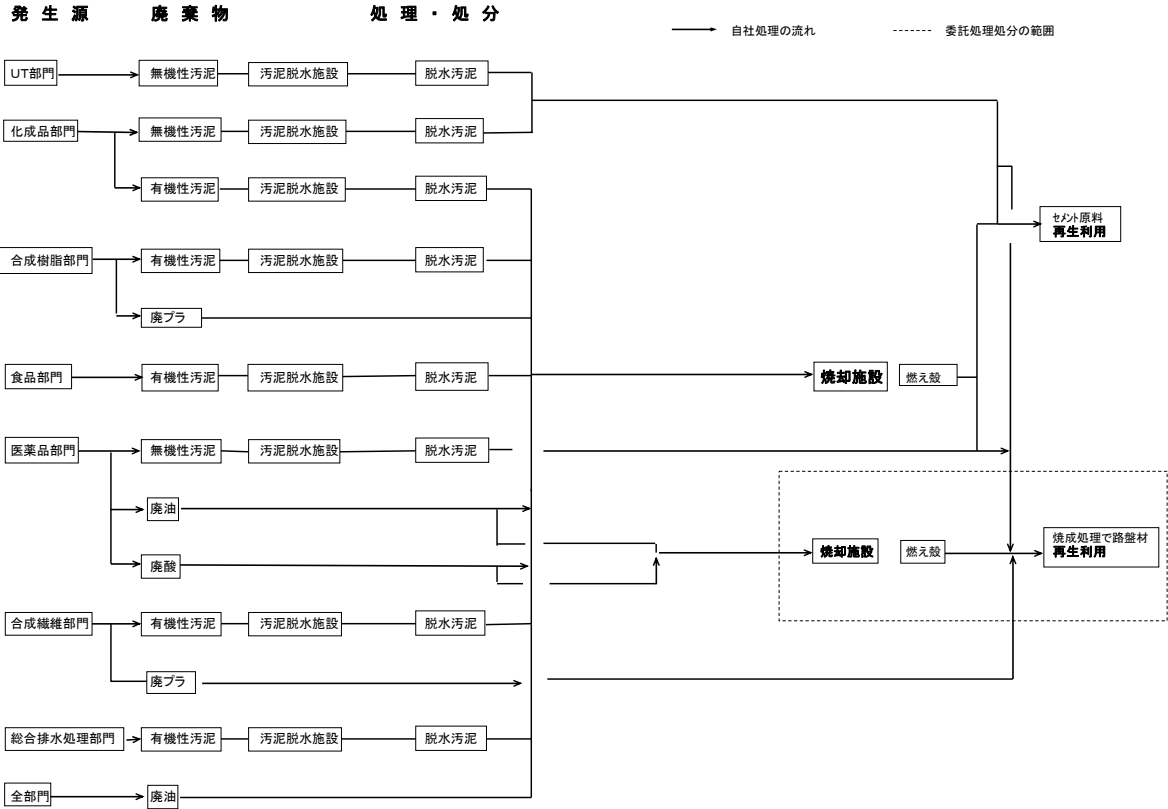
図-3: 廃棄物処理フローシート
