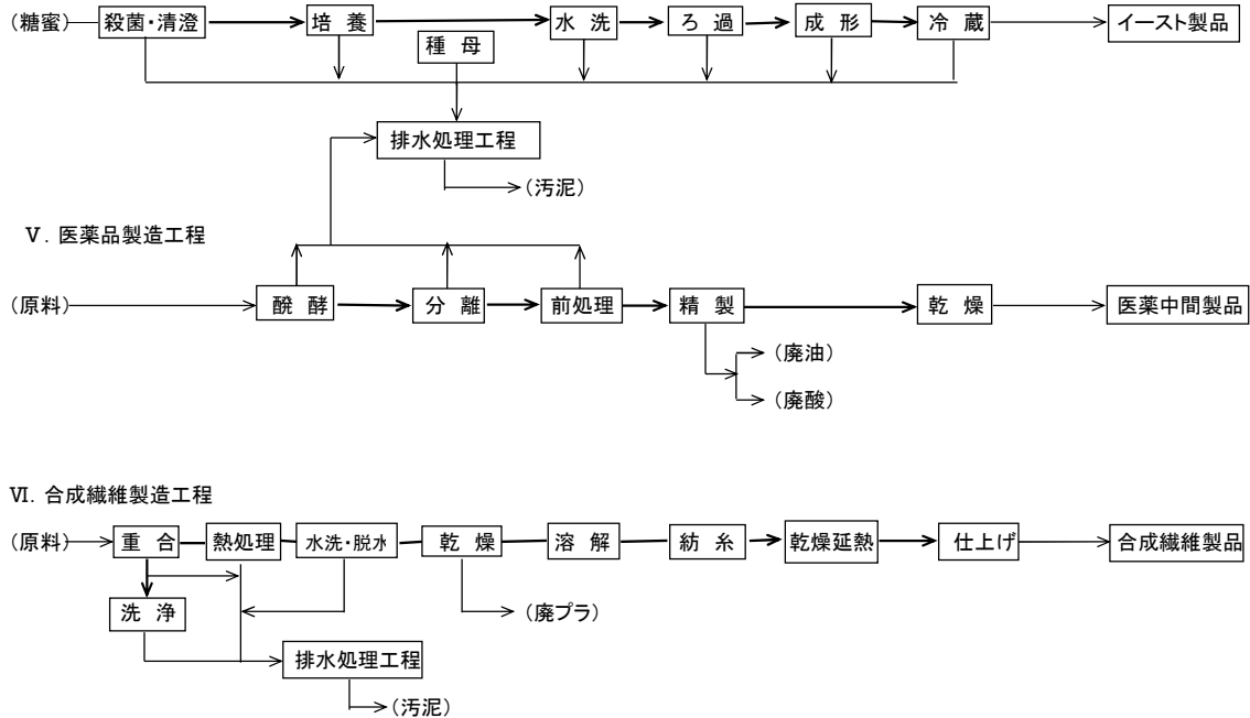
図-2: 製造等フロシートNo.2
