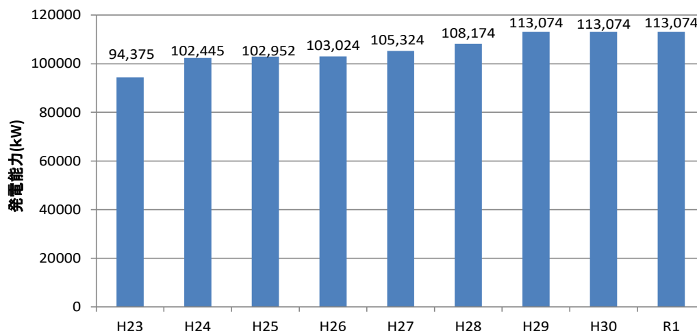
図 17 ごみ処理施設での発電能力
