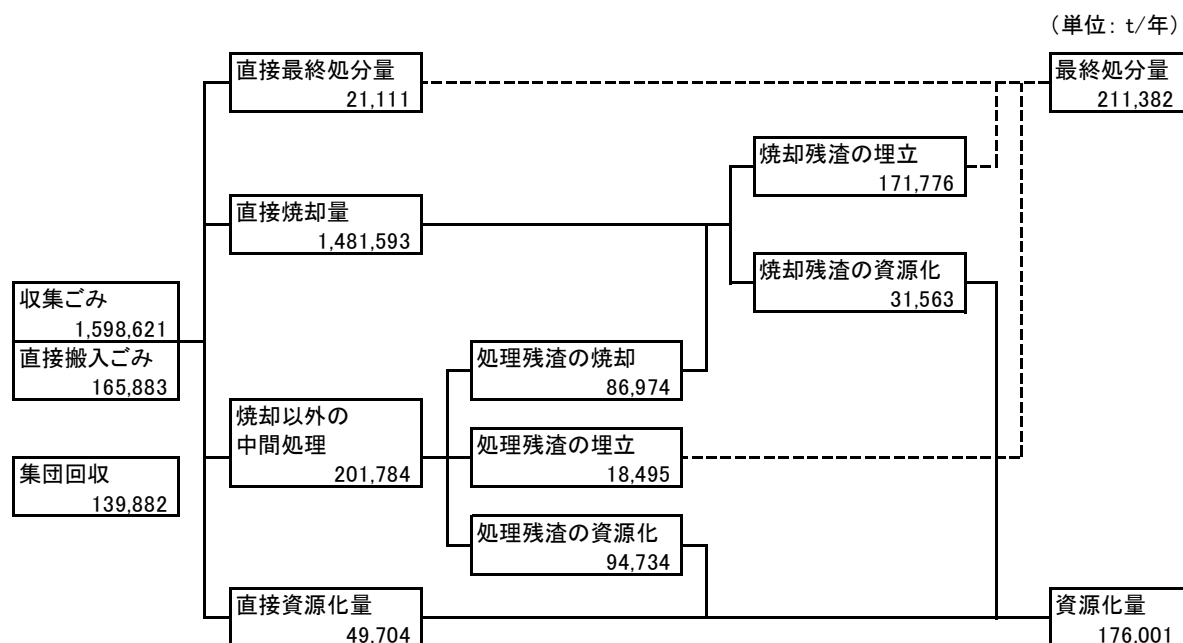
図7 ごみ処理の流れ
