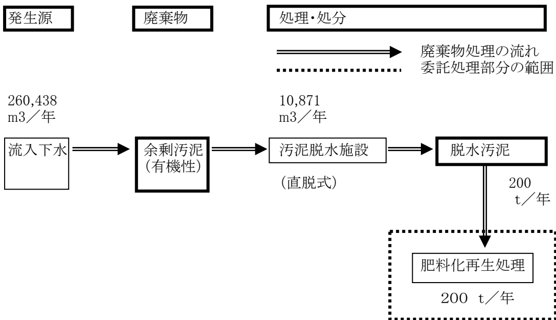
廃棄物処理フロー図(令和3年度実績)
