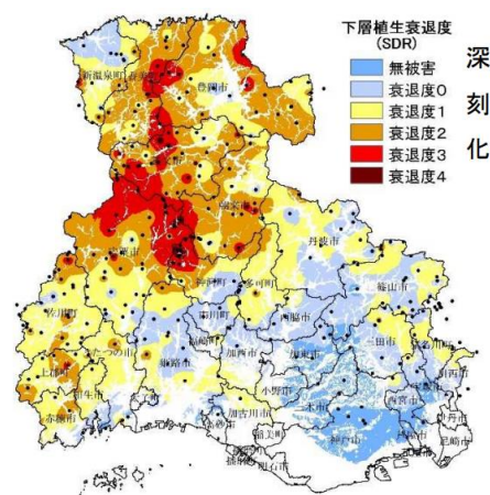
図 2-42 下層植生衰退の状況
