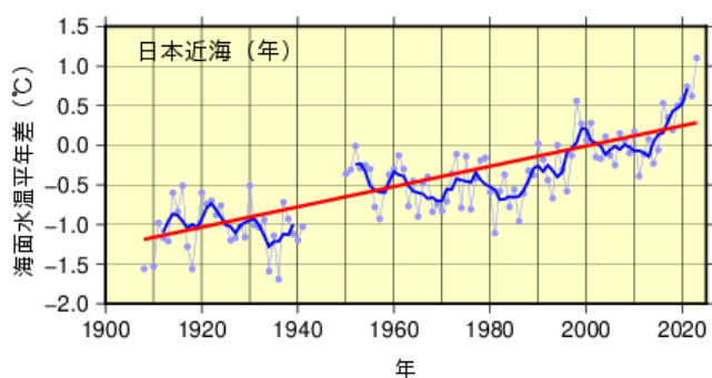
図2-19 日本近海の全海域平均海面水温
