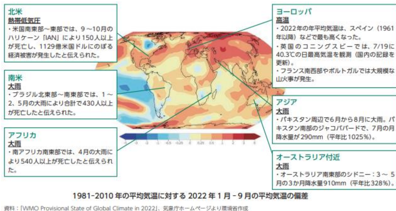
図2-4 2022年の世界各地の異常気象
