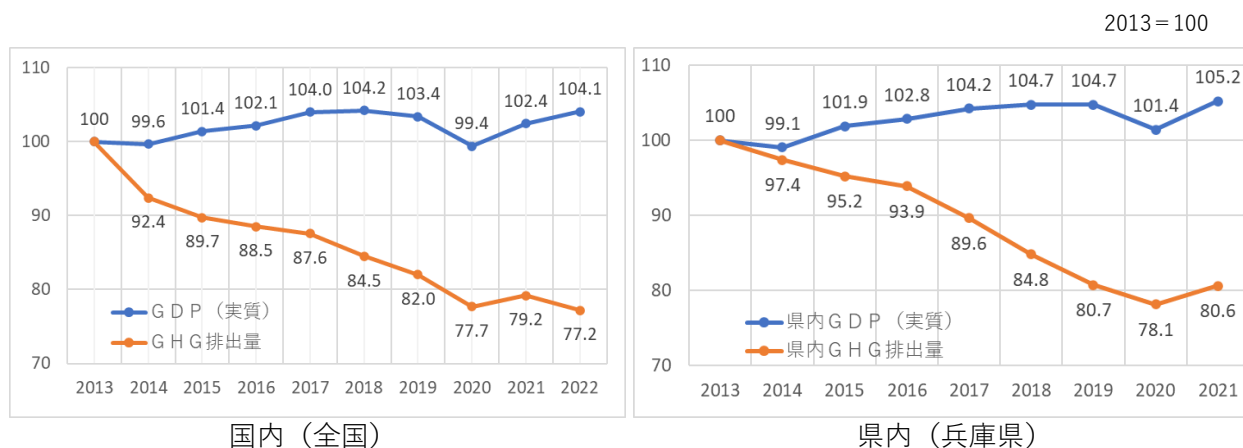
図2-26 国内・県内総生産（GDP）と温室効果ガス（GHG）排出量の推移
