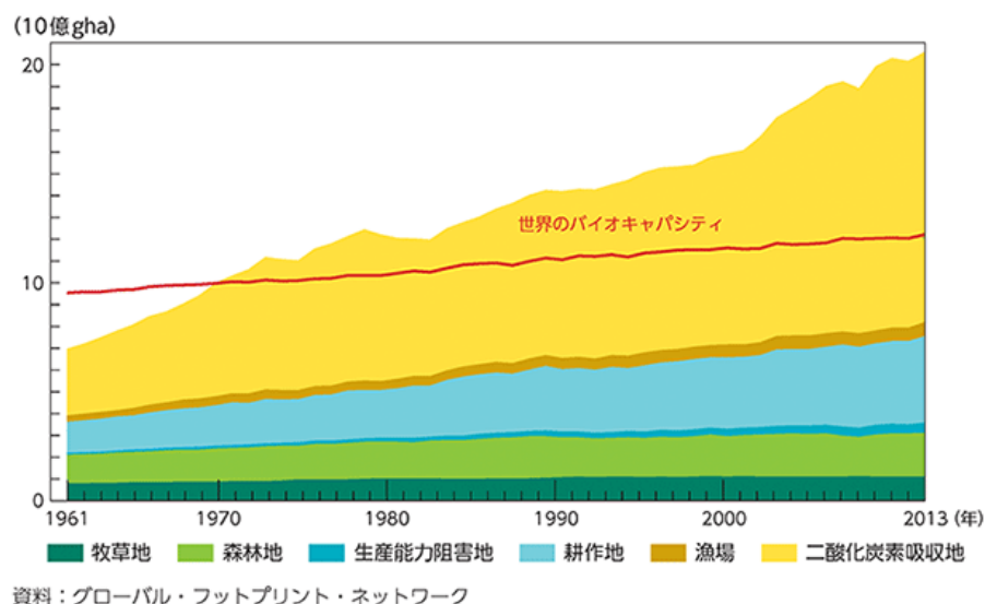
図２－２ 世界のエコロジカル・フットプリントとバイオキャパシティの推移
