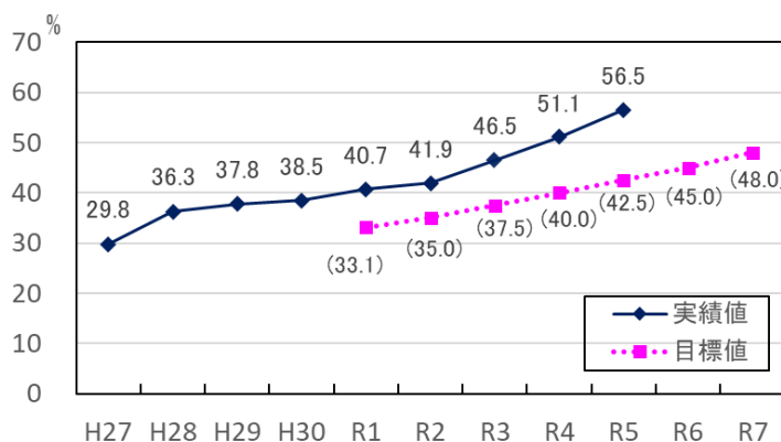
図2-37 新規登録車(乗用車)のうち次世代自動車導入状況 (2023(令和5)年度末)
