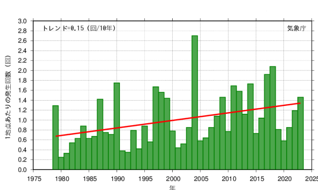
図2-21 兵庫県[7マス]1時間降水量30mm以上（バケをひっくり返したような雨）の年間発生回数 （出典：気象庁ホームページ）
