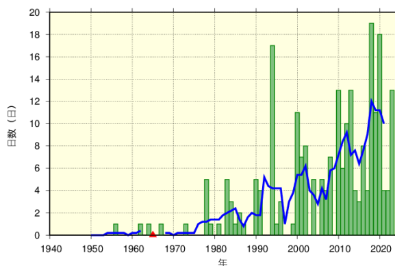
図2-39 姫路の年間猛暑日日数
