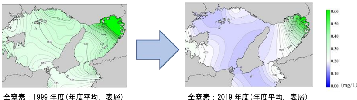
図 2-43 全窒素濃度の推移
