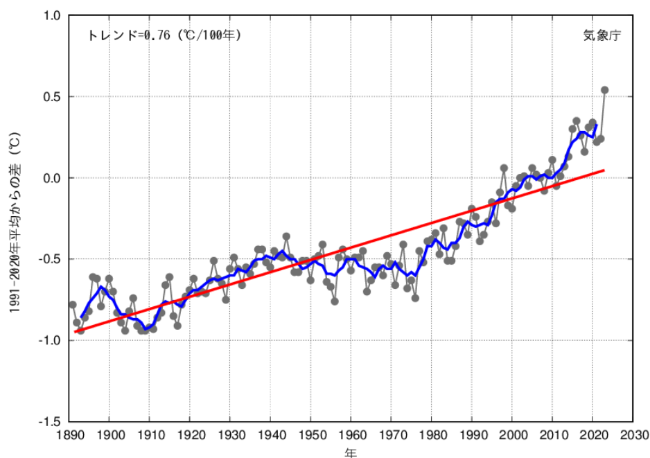
図２－３ 世界の年平均気温偏差
