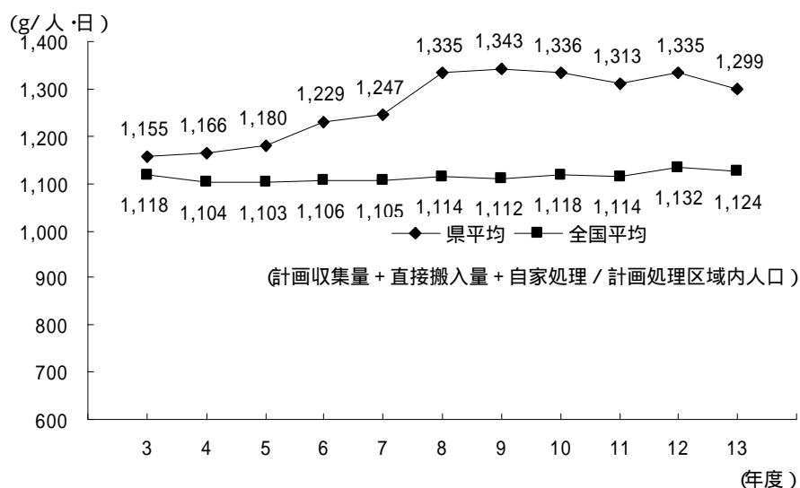
図 - 4 1 人 1 日平均排出量の推移
