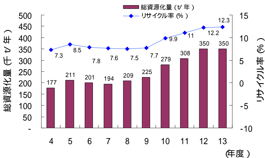
図 - 5 総資源化量とリサイクル率の推移
