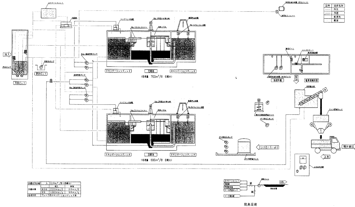
図 1 概略図
