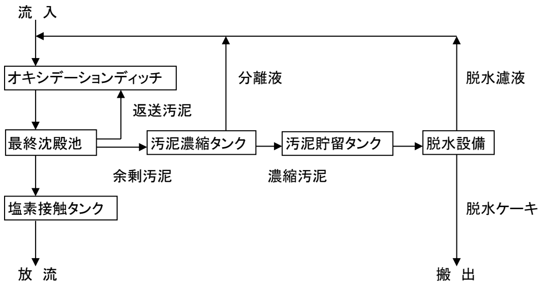
図1 汚水処理工程フローシート
