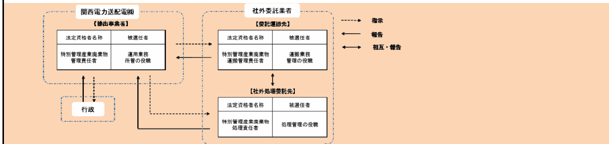
(管理体制図)
