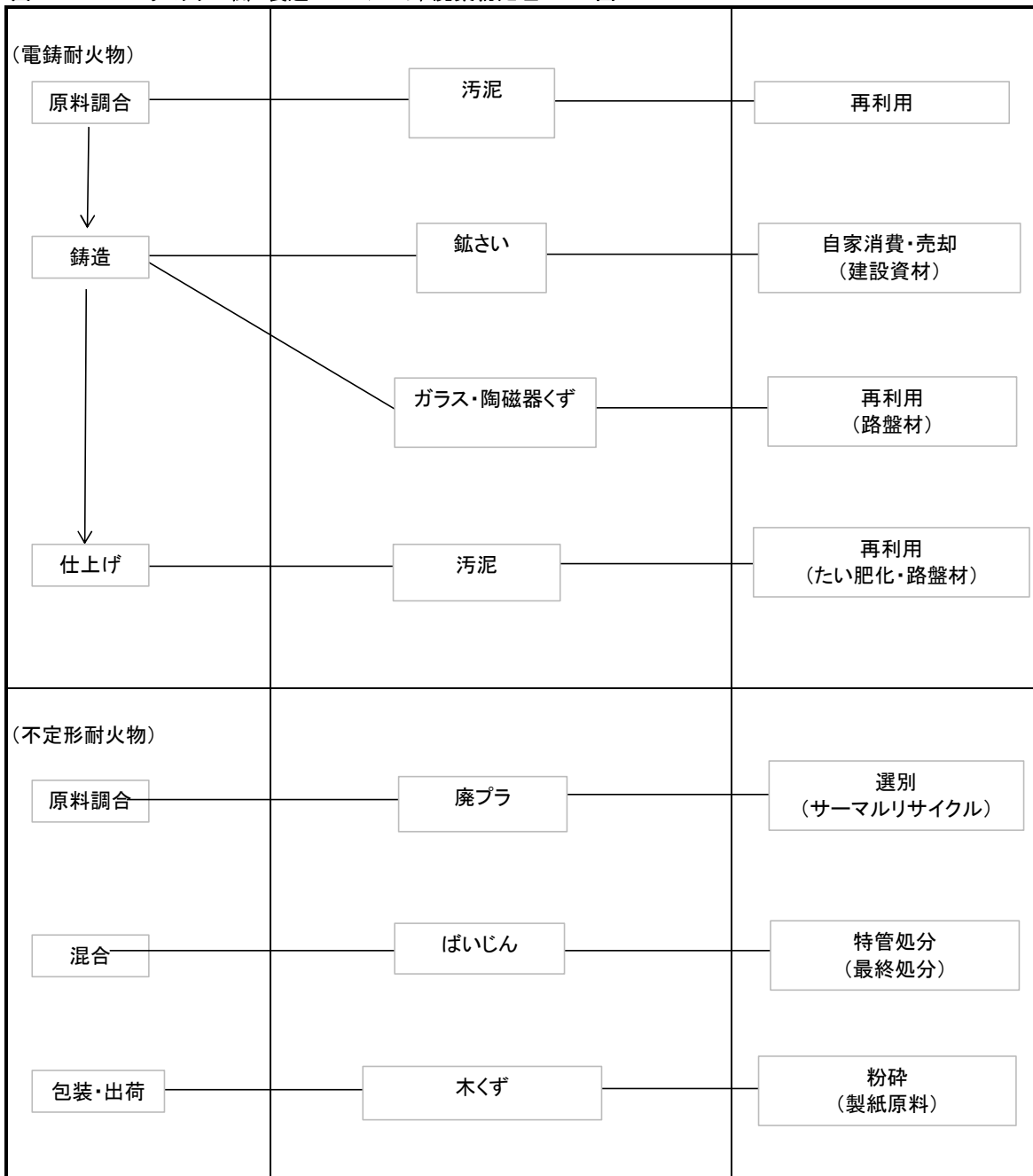
図2 AGCセラミックス㈱ 製造フローシート, 廃棄物処理フロー図
