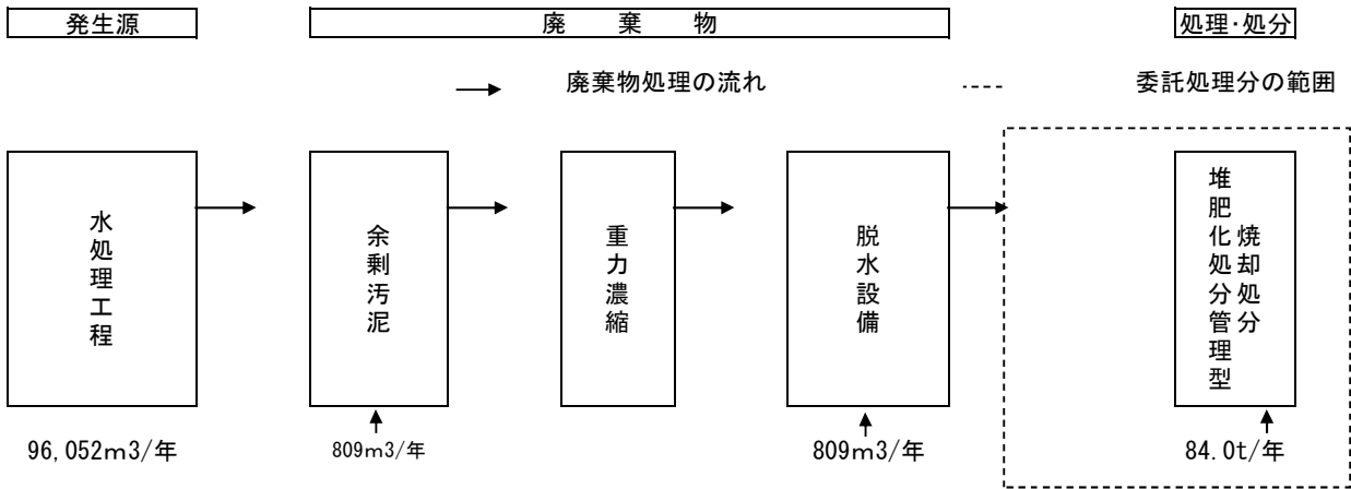
図3 廃棄物処理のフローシート
