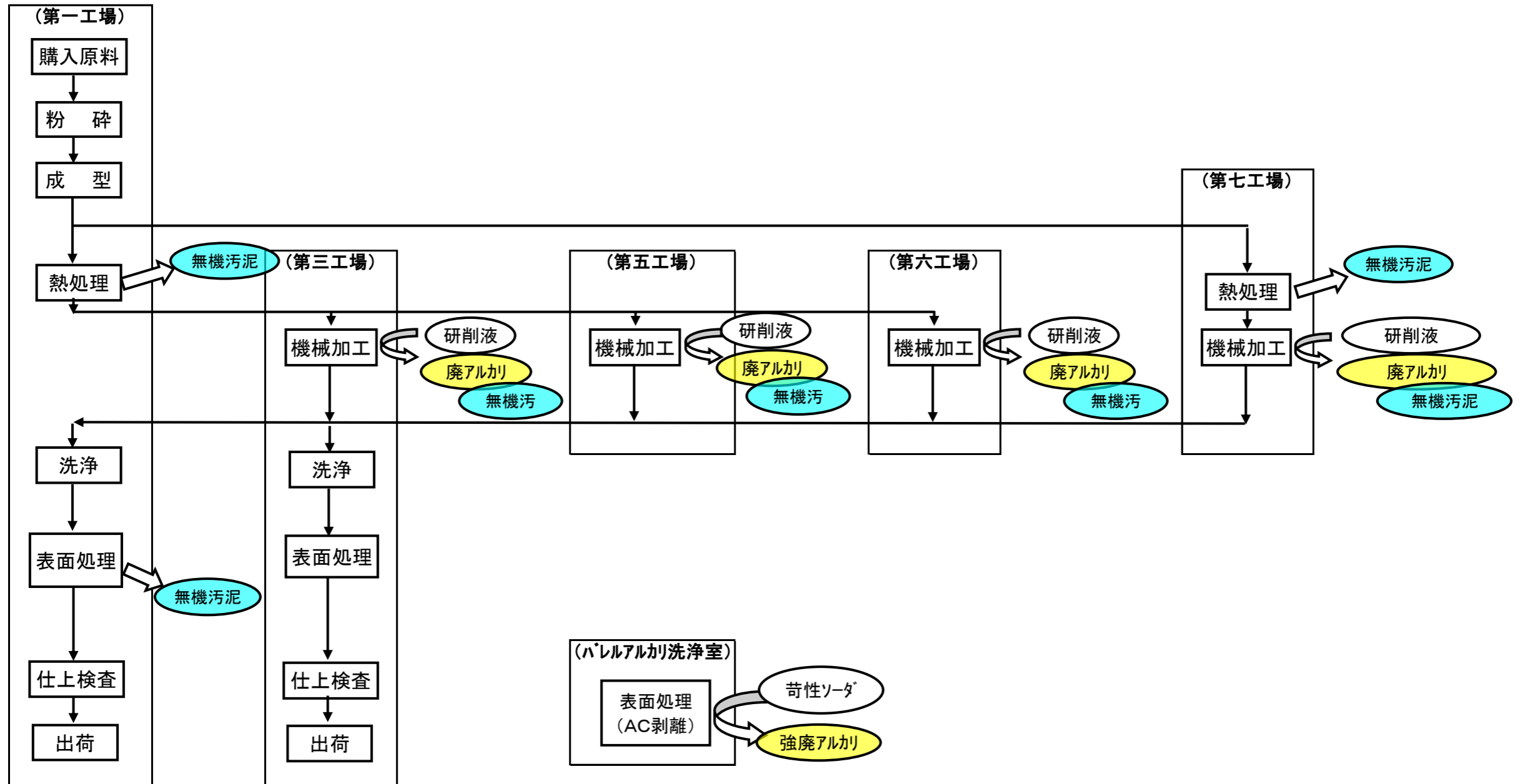
図1 製造工程フロー
