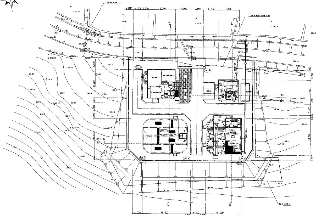
配置図 1/250
