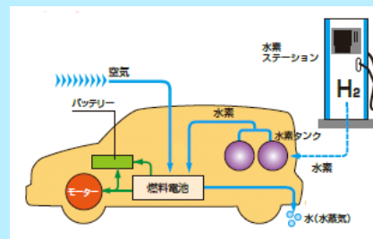
FCVの仕組み
