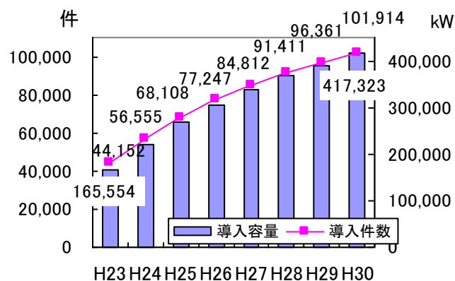
図3-1-5 県内の住宅用太陽光発電システム 導入件数及び容量(累計)
