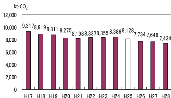
図3-1-12 運輸部門の温室効果ガス排出量
