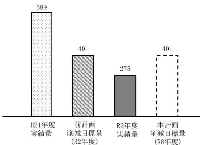
図2-2 自動車排出粒子状物質の総排出量（対策地域）の状況（t／年）
