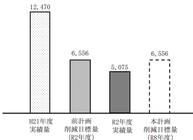
図2-1 自動車排出窒素酸化物の総排出量（対策地域）の状況（t／年）
