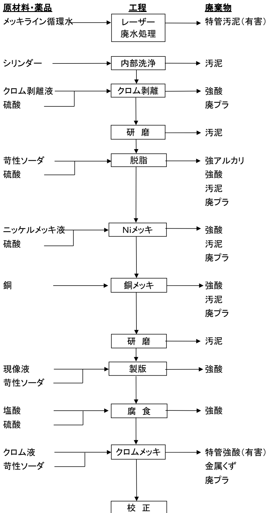
図 2 製造等フローシート及び廃棄物発生フロー図 (製版)
