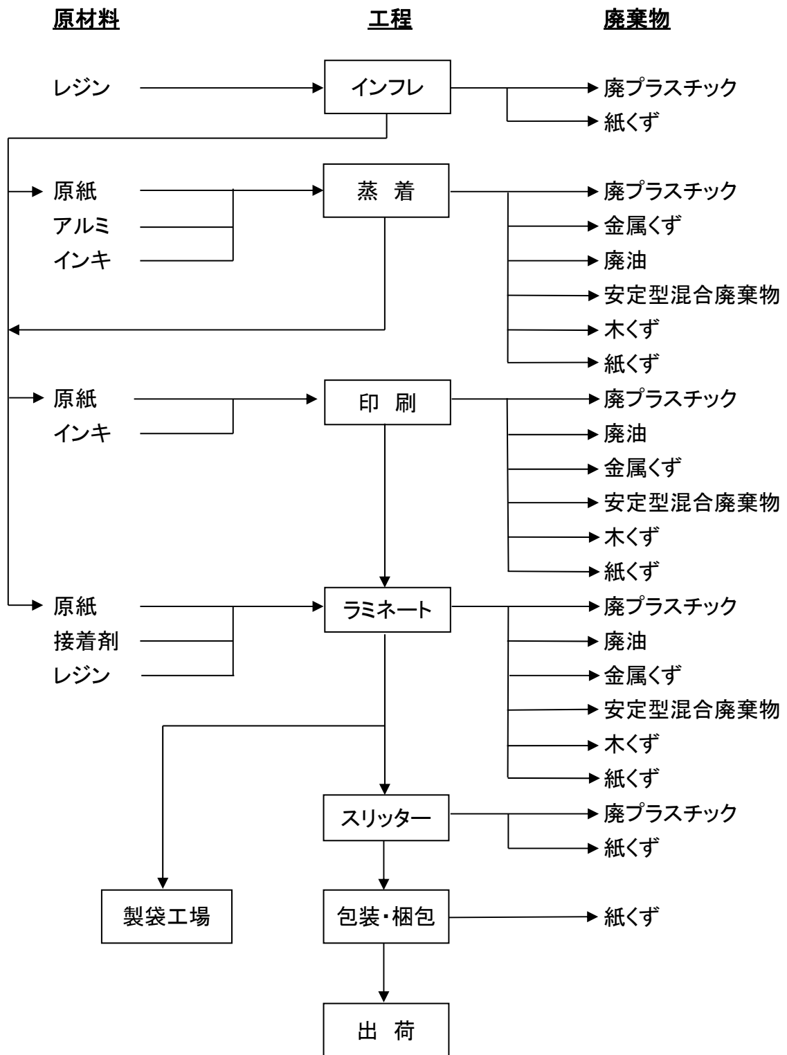
図 1 製造等フローシート及び廃棄物発生フロー図 (印刷、ラミネート、蒸着、インフレ、スリッター)
