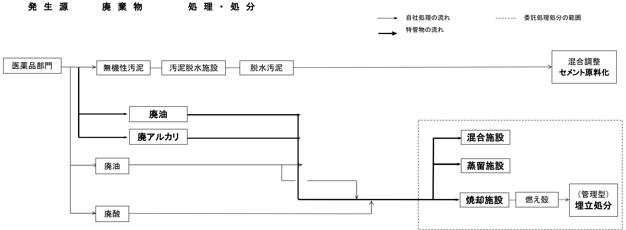
図-2: 特別管理産業廃棄物処理フローシート
