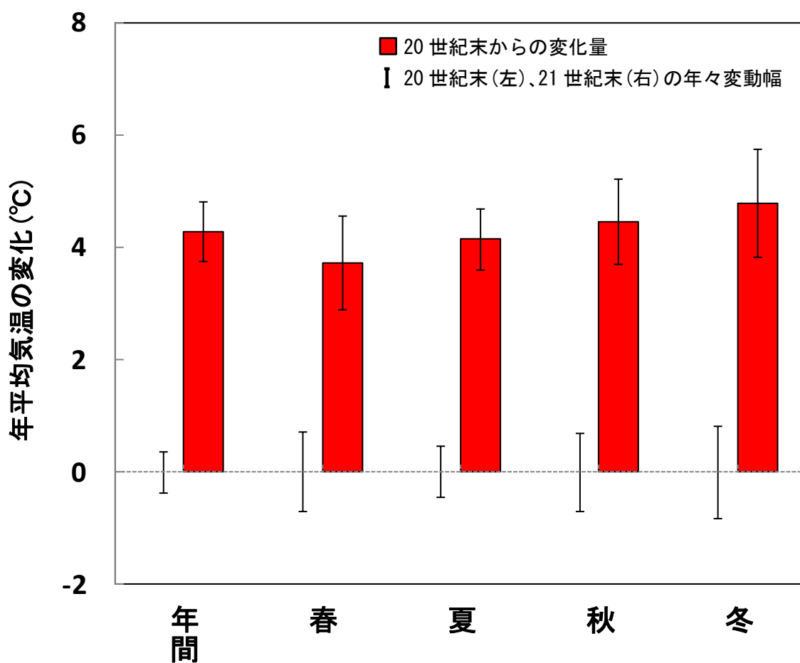
県内の年平均気温の将来予測
