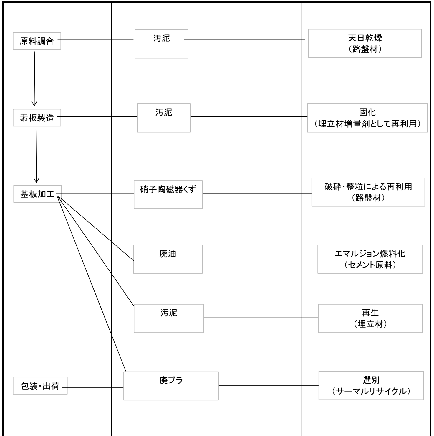
図1 旭硝子(株)高砂工場 製造フローシート, 廃棄物処理フロー図
