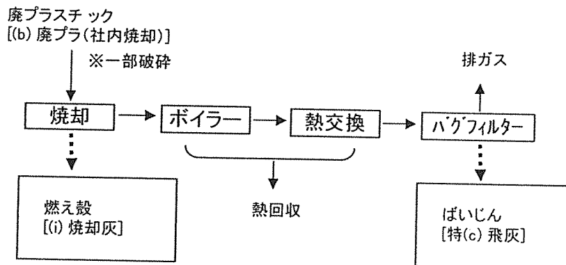
図4 焼却処理 フローシート [NO.4]
