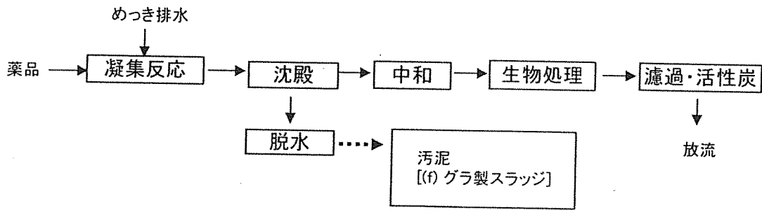
図3 めっき排水処理 フローシート [NO.3]
