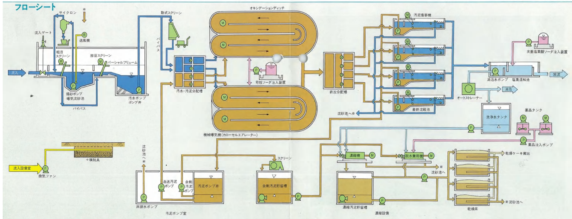
オキシデーションディッチ
