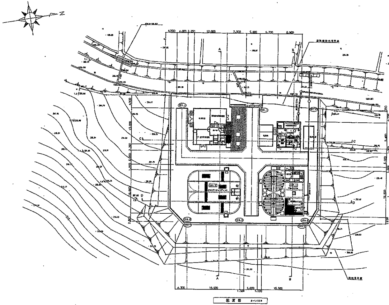
配置図 8-1/110
