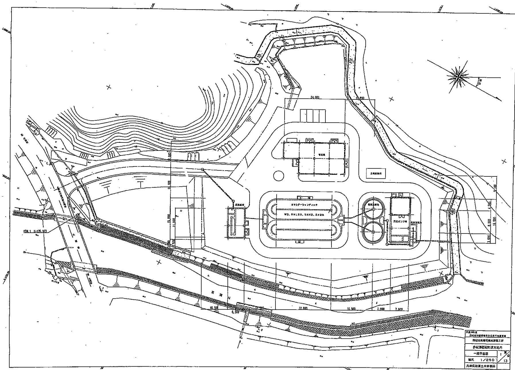
図2 処理場配置図
