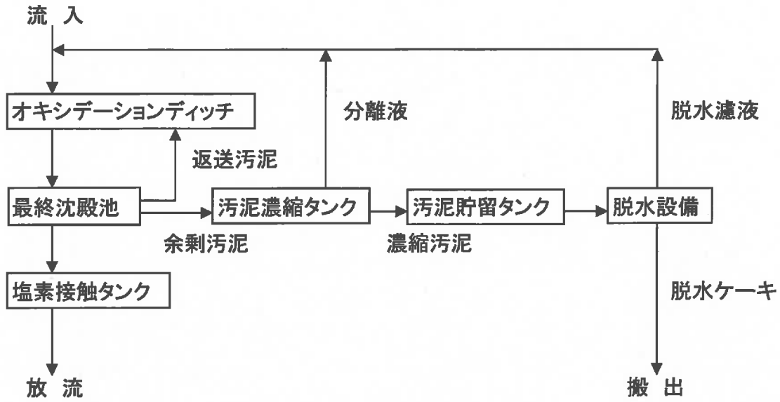
図1 汚水処理工程フローシート
