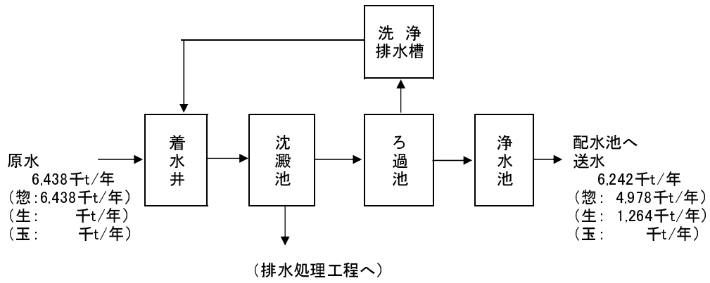
図 1 浄水製造フローシート
