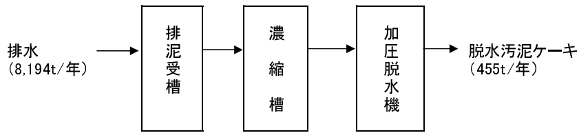
図 2 排水処理フローシート
