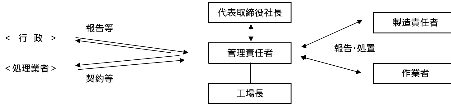
(管理体制図)
