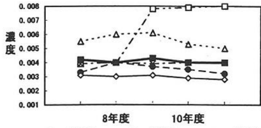
ニッケル濃度の経年変化 播磨地域 ( \mu\text{g}/\text{m}^3 )
