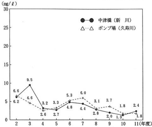
第2-2-24図 主要測定点におけるBOD75%値の経年変化 〔阪神地区都市河川〕
