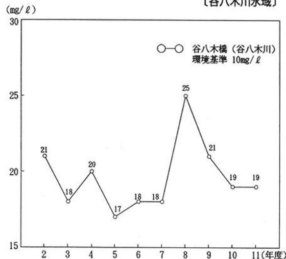
第2-2-18図 環境基準点におけるBOD75%値の経年変化 〔谷八木川水域〕
