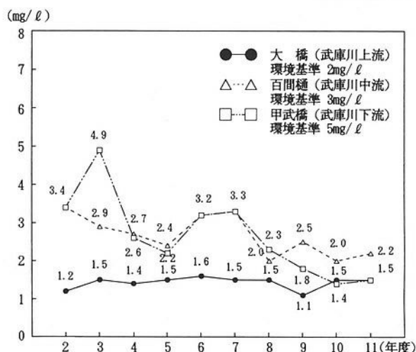
第2-2-11図 環境基準点におけるBOD75%値の経年変化 〔武庫川水域〕
