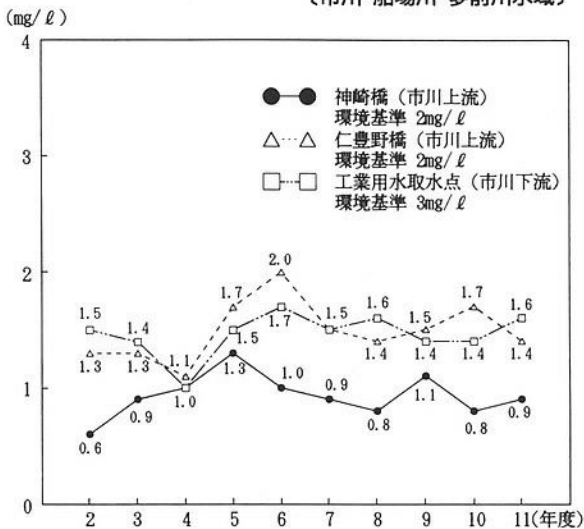
第2-2-14図 環境基準点におけるBOD75%値の経年変化 〔市川・船場川・夢前川水域〕
