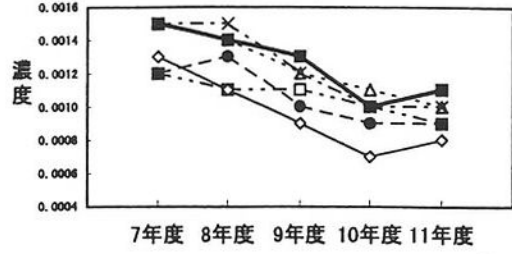
カドミウム濃度の経年変化 播磨地域 ( \mu\text{g}/\text{m}^3 )
