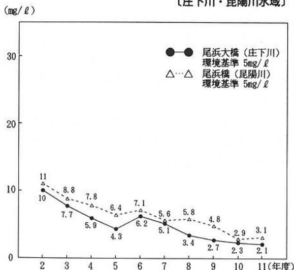
第2-2-20図 環境基準点におけるBOD75%値の経年変化 〔庄下川・昆陽川水域〕
