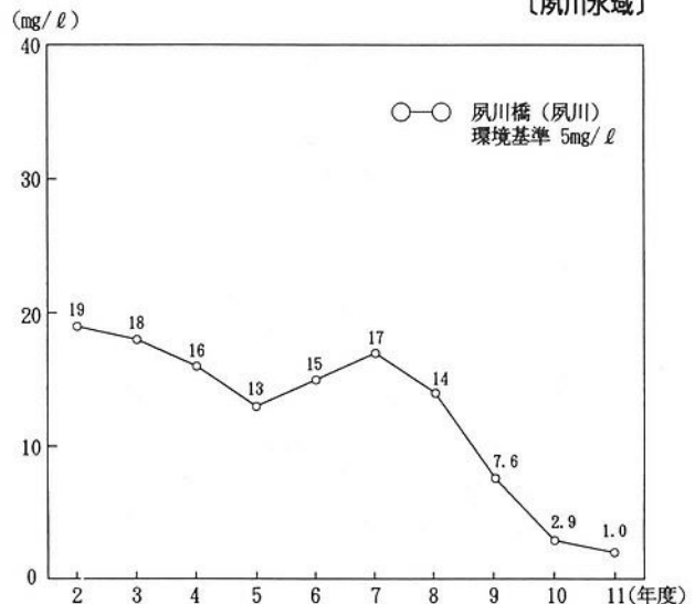
第2-2-21図 環境基準点におけるBOD75%値の経年変化 〔夙川水域〕
