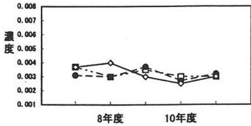
ニッケル濃度の経年変化 阪神地域 ( \mu\text{g}/\text{m}^3 )
