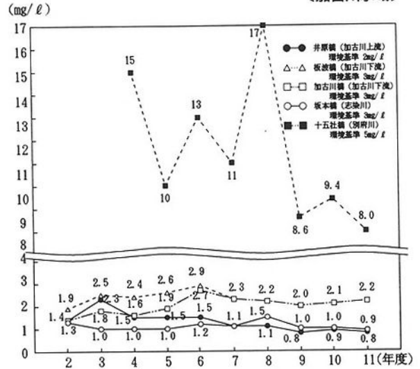
第2-2-13図 環境基準点におけるBOD75%値の経年変化 (加古川水域)
