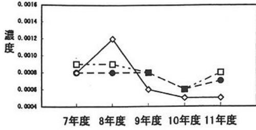
カドミウム濃度の経年変化 阪神地域 ( \mu\text{g}/\text{m}^3 )
