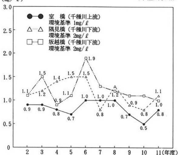
第2-2-16図 環境基準点におけるBOD75%値の経年変化 〔千種川水域〕
