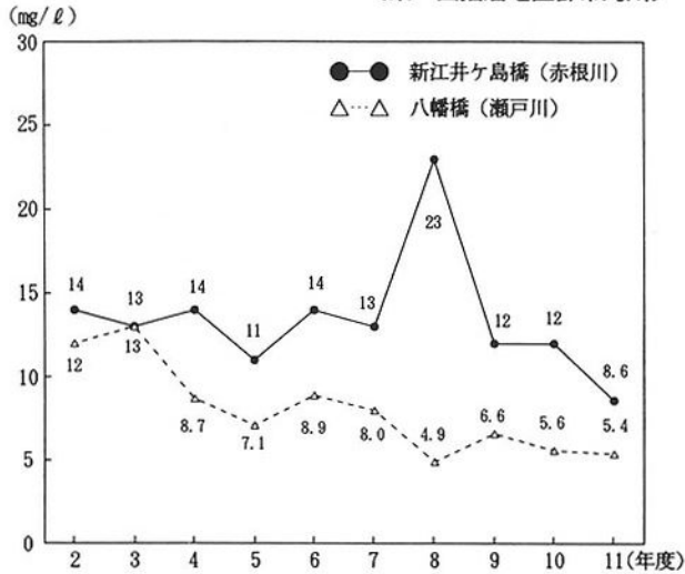
第2-2-26図 主要測定点におけるBOD75%値の経年変化 〔東・西播磨地区都市河川〕
