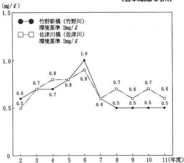
第2-2-23図 環境基準点におけるBOD75%値の経年変化 (日本海流入河川)
