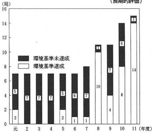
第2-2-39図 浮遊粒子状物質の環境基準達成状況 (長期的評価)
