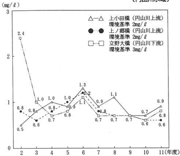
第2-2-22図 環境基準点におけるBOD75%値の経年変化 (円山川水域)
