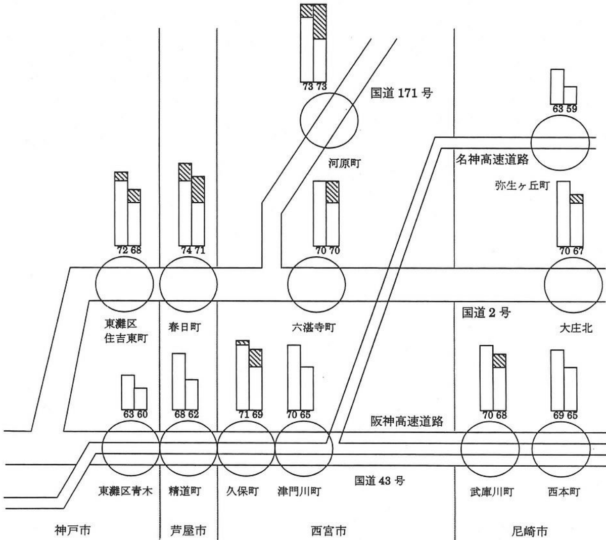
第2-2-43図 阪神臨海部における自動車騒音の現況
