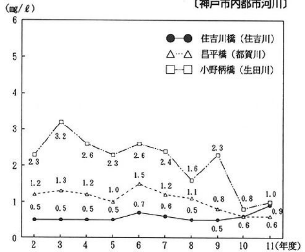
第2-2-25図 主要測定点におけるBOD75%値の経年変化 〔神戸市内都市河川〕
