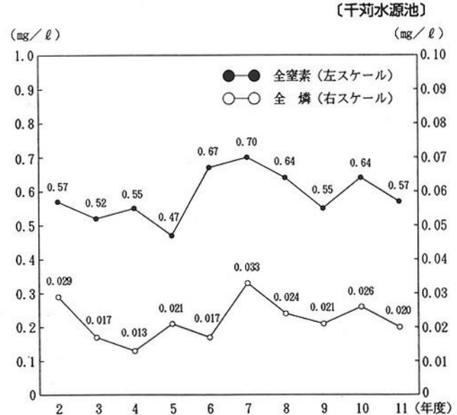
第2-2-29図 全窒素、全磷(全層平均値)の経年変化
