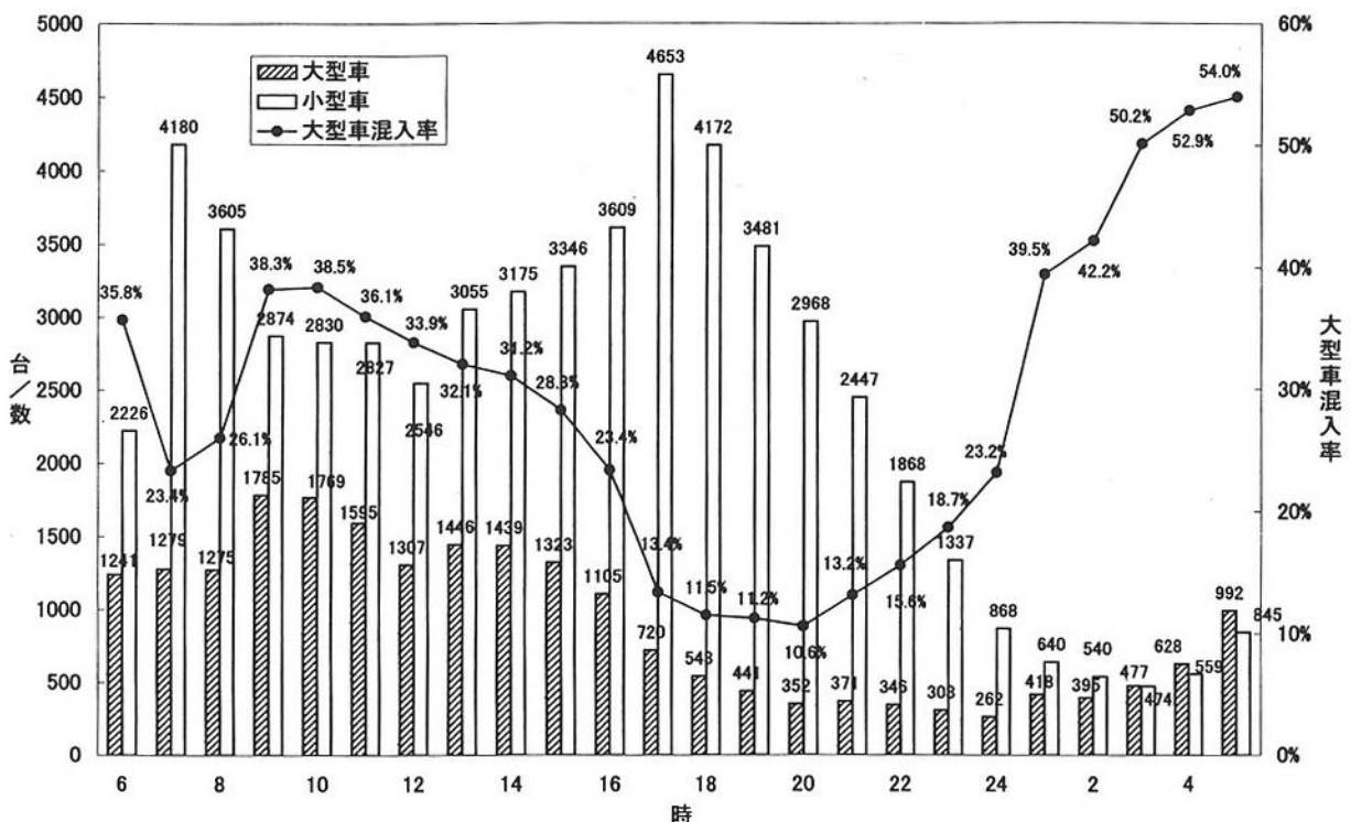
第2-2-44図 国道43号の芦屋地域における交通量の経時変化と大型車混入率
