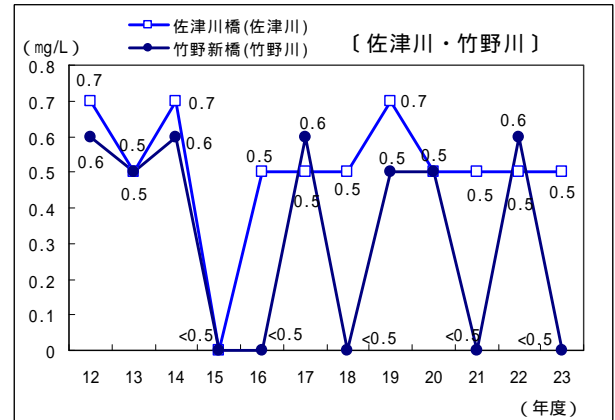
第1-14 図 環境基準点における BOD75%値の経年変化
