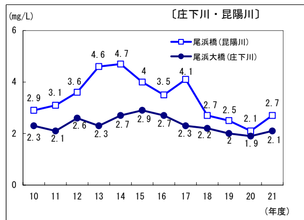
第7-2-2 図 環境基準点におけるBOD75%値の経年変化
