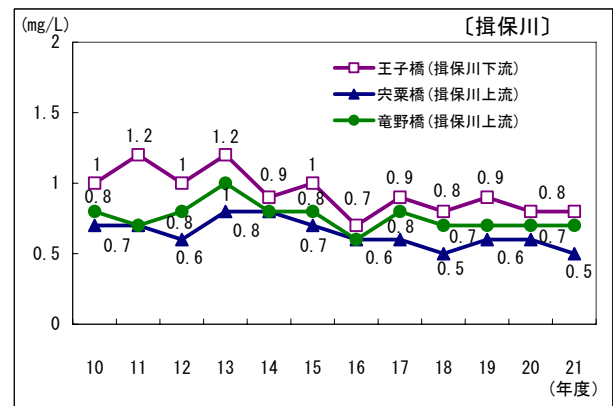
第7-2-11図 環境基準点におけるBOD75%値の経年変化
