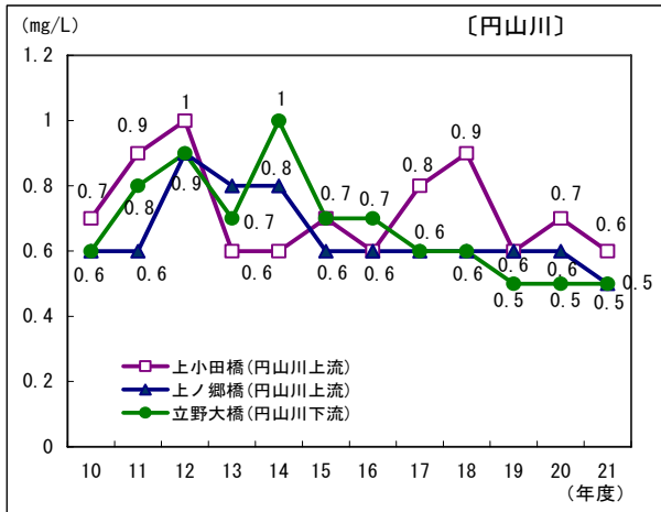
第7-2-13図 環境基準点におけるBOD75%値の経年変化
