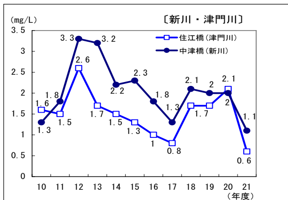
第7-2-15図 環境基準点におけるBOD75%値の経年変化
