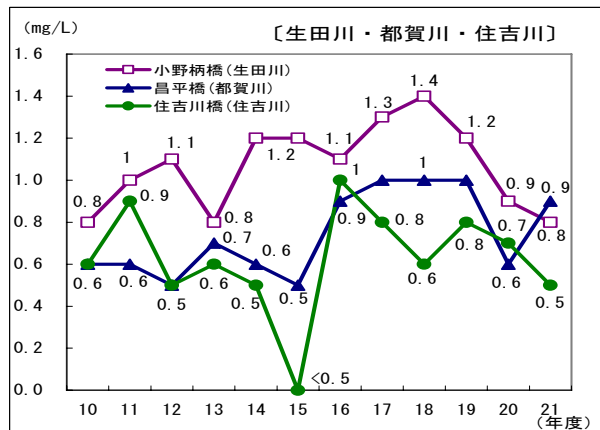
第7-2-16図 主要測定点におけるBOD75%値の経年変化
