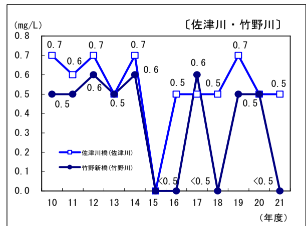
第7-2-14図 環境基準点におけるBOD75%値の経年変化
