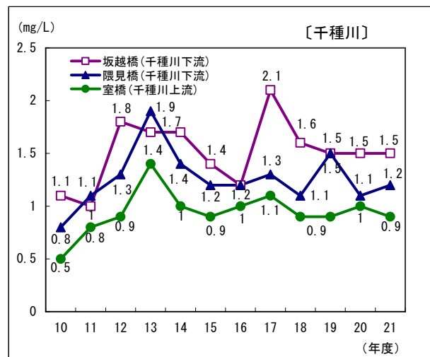
第7-2-12図 環境基準点におけるBOD75%値の経年変化
