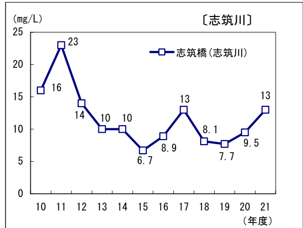
第7-2-18図 主要測定点におけるBOD75%値の経年変化
