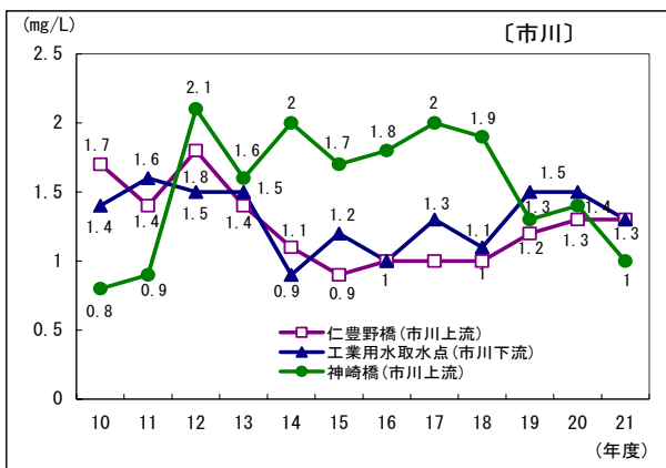
第7-2-10図 環境基準点におけるBOD75%値の経年変化
