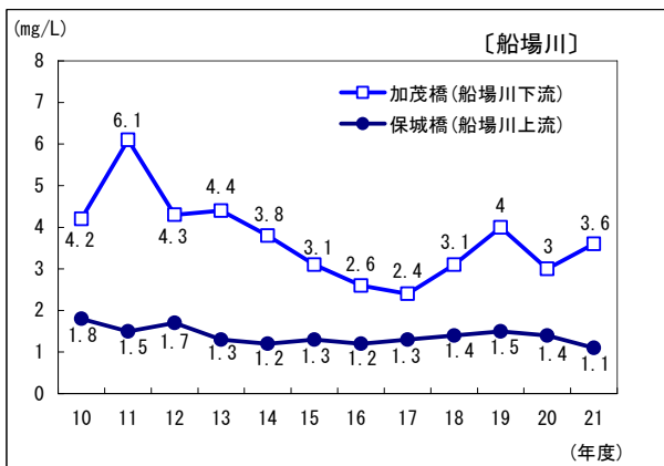
第7-2-12図 環境基準点におけるBOD75%値の経年変化
