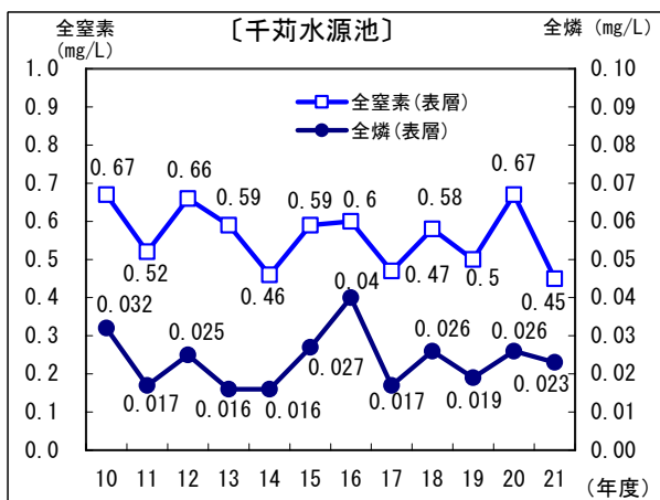
第7-2-20図 全窒素・全りん（表層平均値）の経年変化
