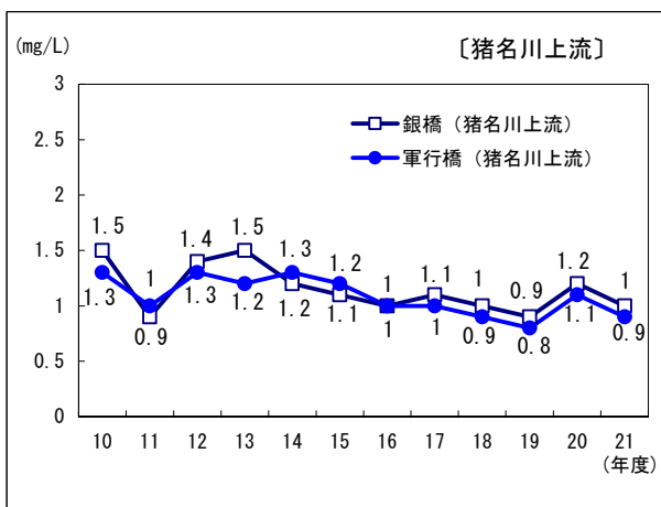
第7-2-1 図 環境基準点におけるBOD75%値の経年変化
