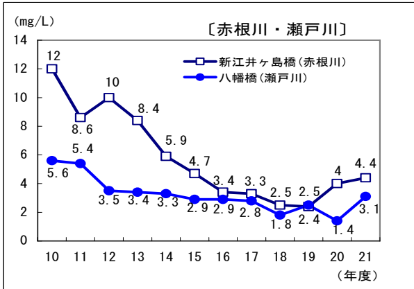
第7-2-17図 主要測定点におけるBOD75%値の経年変化
