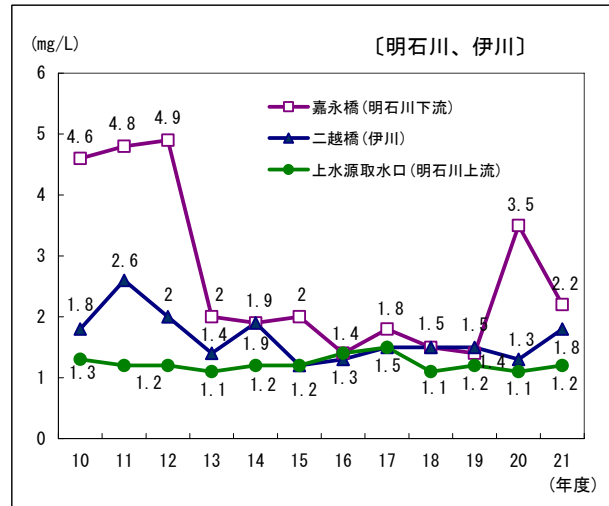
第7-2-6図 環境基準点におけるBOD75%値の経年変化
