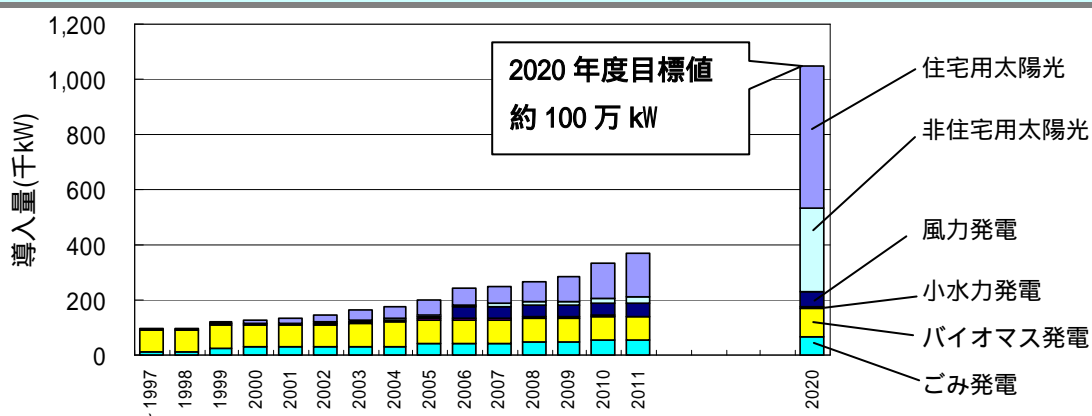
図5 兵庫県内の再生可能エネルギー導入量の推移及び2020年度導入目標
